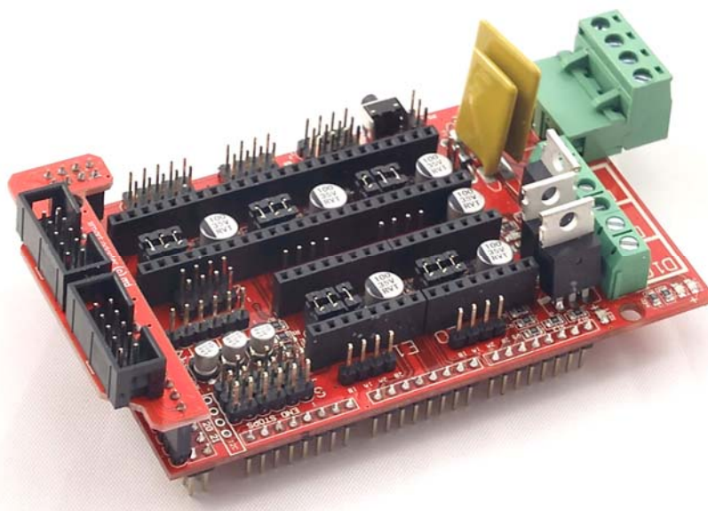
Rysunek 5.28 RAMPS 1.4
