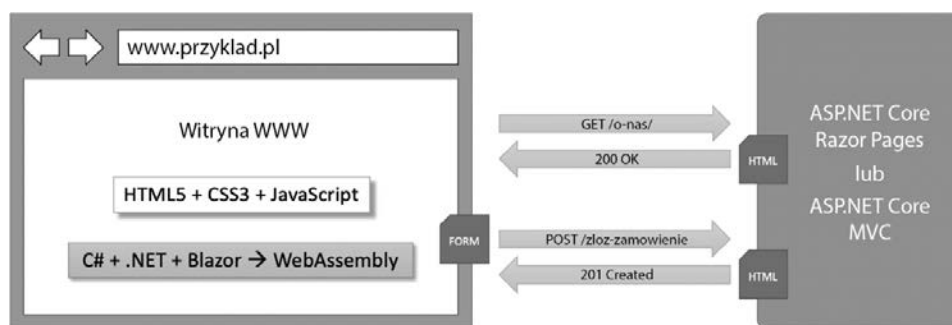
Rysunek 12.1. Sposób użycia języka C# i środowiska .NET do tworzenia serwisów sieciowych po stronie serwera i po stronie klienta
