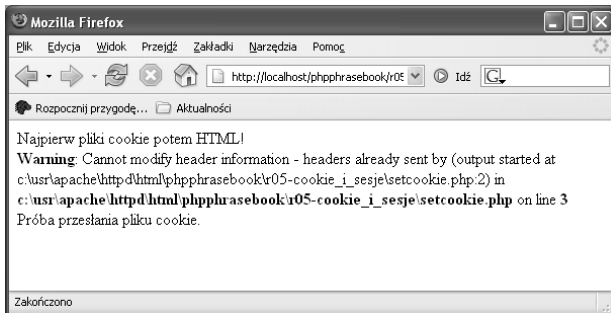
Rysunek 5.3. Pliki cookie trzeba przesać przed wysłaniem zawartości HTML
