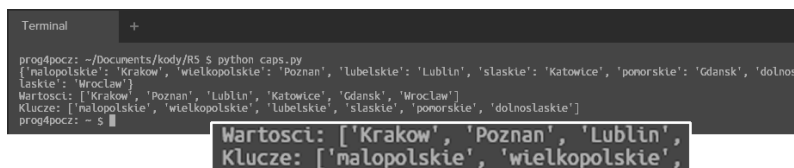
Rysunek 5.7. Wyniki przedstawiające zastosowanie dwóch funkcji słowników: values() i keys()
